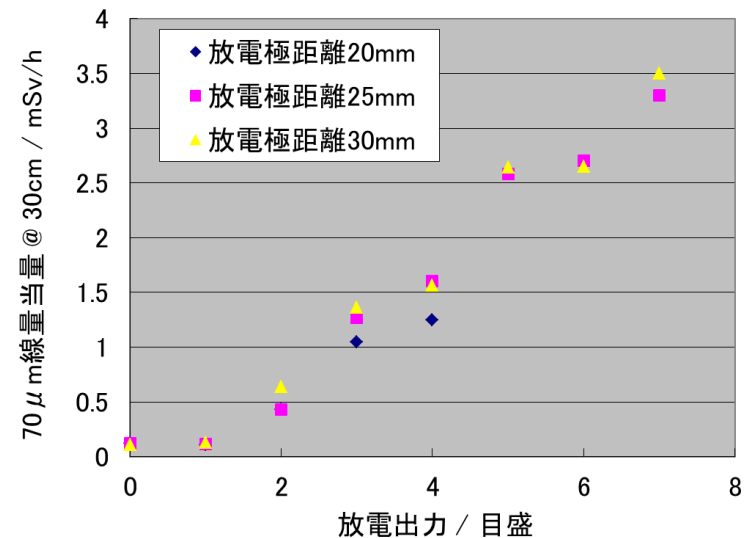
放電出力と70 \mu m線量当量 30cmの相関
