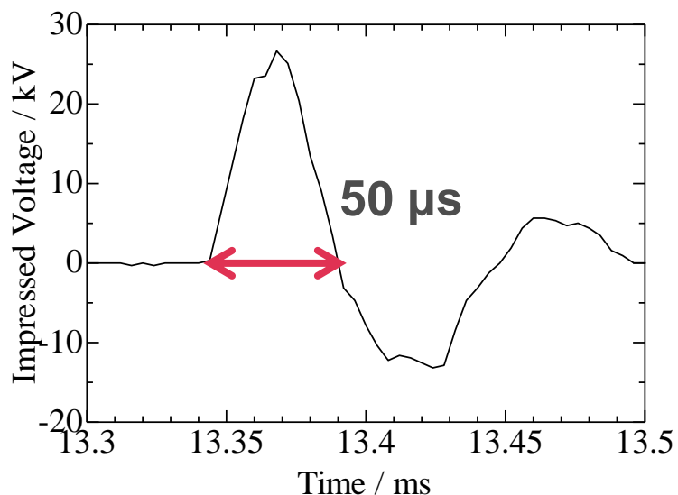
誘導コイルから出力される高電圧パルス
