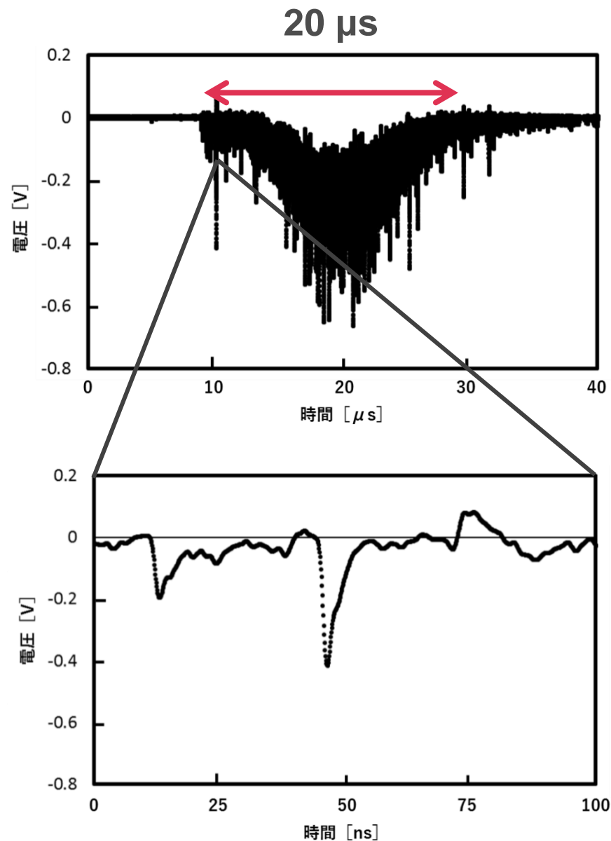
クルックス管由来のX線を計測した結果
