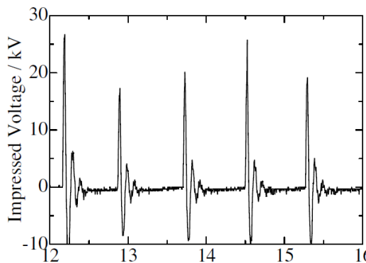
放電極距離 20mm 放電出力 3 電流 75 \mu\text{A} , 線量率 1.05\text{mSv/h}
