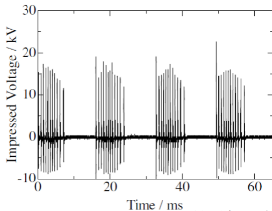
放電極距離 20mm 放電出力 0 電流 40 \mu\text{A} , 線量率 120 \mu\text{Sv/h}
